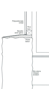
DÉTAIL 3 Fermeture ouest
